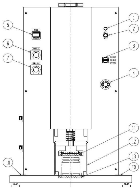
正面図
